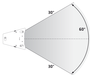
Abb.: 2 Horizontale Abstrahlung
