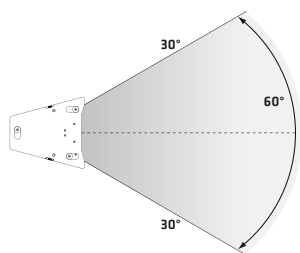
Fig. 2 Dispersion horizontale
