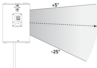
Fig.: 1 Fascio di luce verticale
