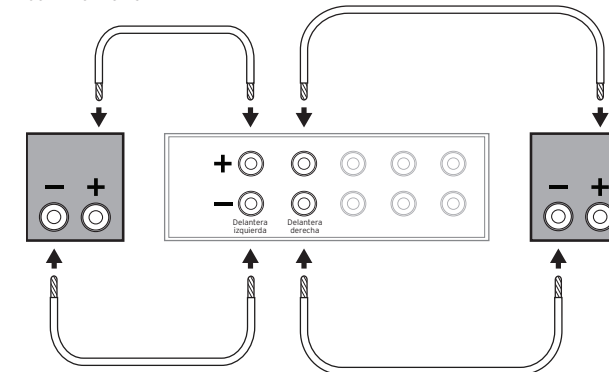
FIGURA 3 CONEXIONES ESTÁNDAR
