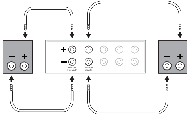
FIGURA 3 CONEXÕES PADRÃO
