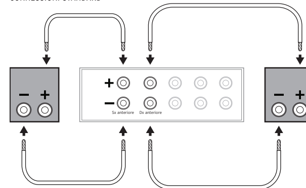
FIGURA 3 CONNESSIONI STANDARD
