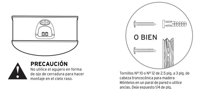
FIGURA 4 MONTAJE DE LOS ALTAVOCES SURROUND EN LA PARED
