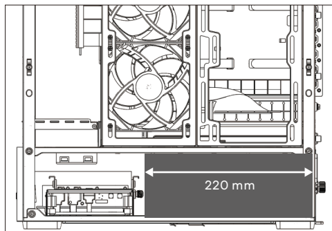
PSU clearance/PSU長度限制/Dégagement PSU
