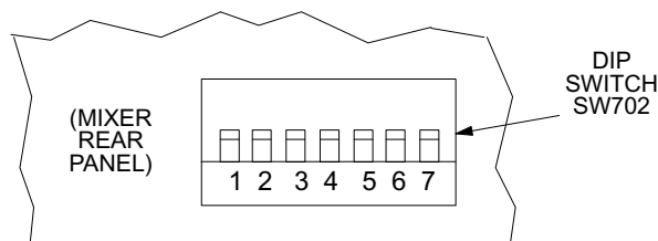
FIGURE 3 FONCTIONS DE L'INTERRUPTEUR À POSITIONS MULTIPLES SW702
